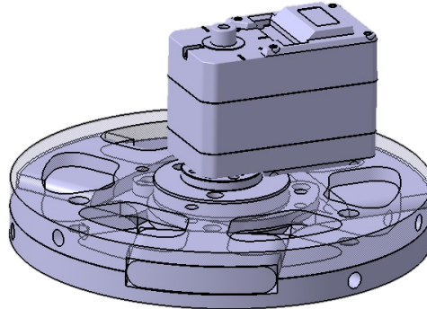
FIGURE 4.3 – Système d'aérofrein d'SP-02 sur CATIA
