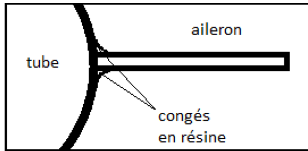
FIGURE 4.2 – Procédé de collage ailerons/structure avec congés en résine
