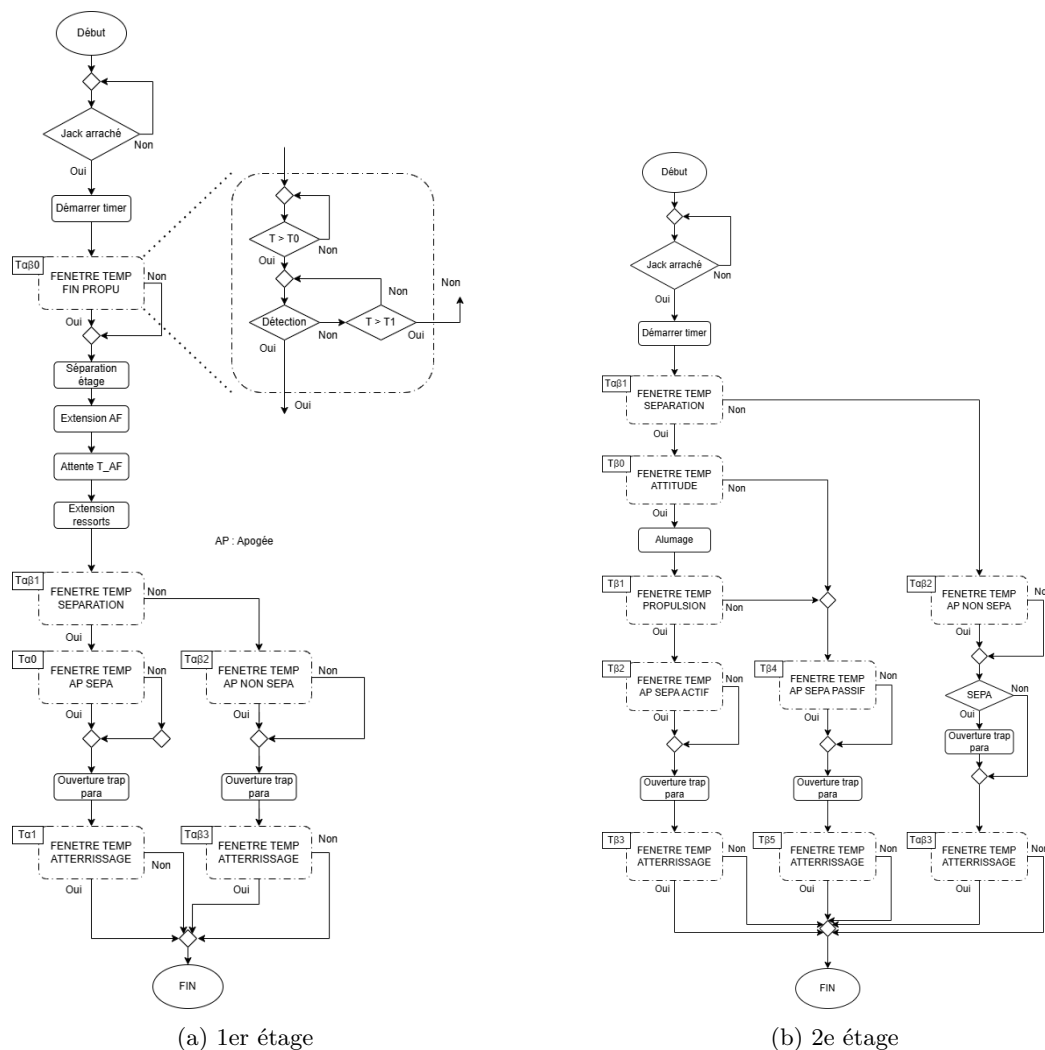
FIGURE 5.1 – Schémas fonctionnels des séquenceurs des deux étages
