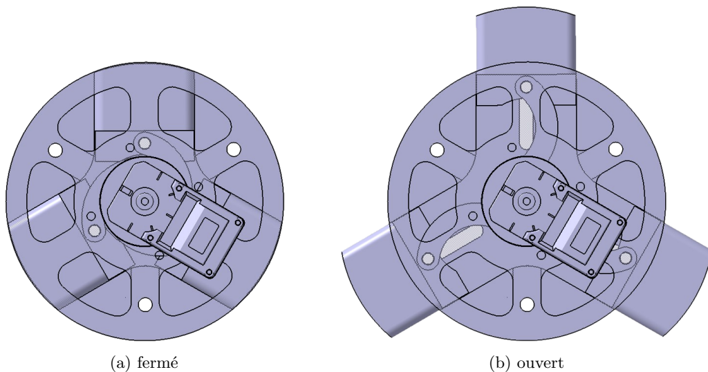
FIGURE 4.4 – Position des aérofreins d'SP-02
