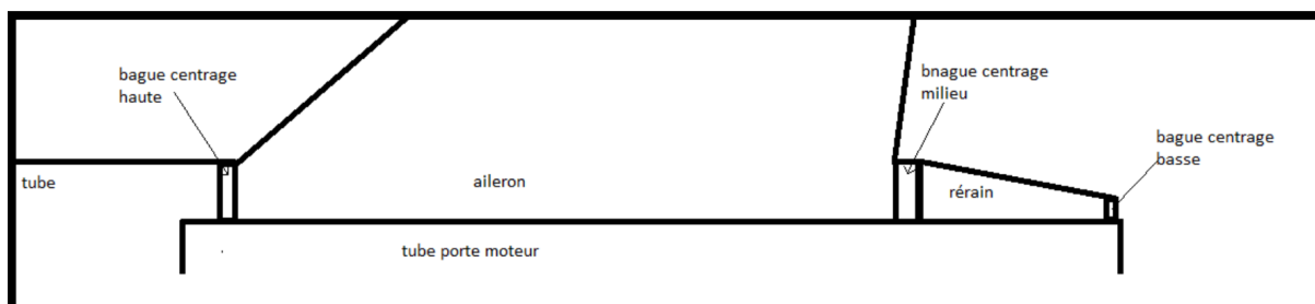
FIGURE 4.1 – Procédé de collage ailerons/tube porte-moteur
